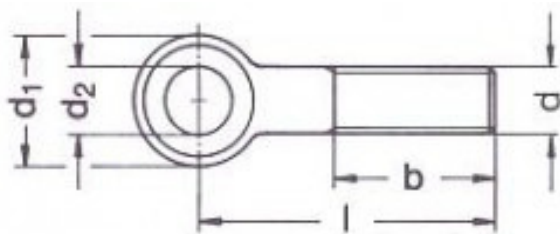
EYE BOLT ( DIN-444 )
